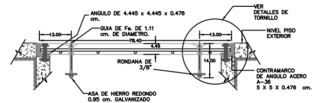
DETALLE TAPA: CORTE C-C'
