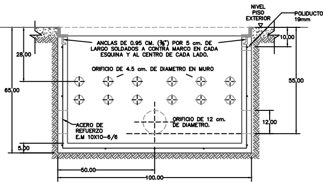
CORTE A-A'
