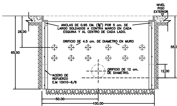
CORTE A-A'
