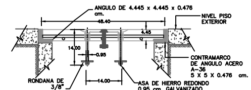
DETALLE TAPA: CORTE D-D'
